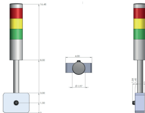
Figura 7. Dimensiones del dispositivo de medición
