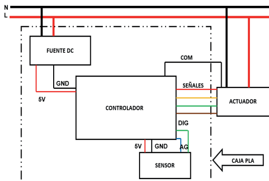
Figura 8. Diagrama de conexión
