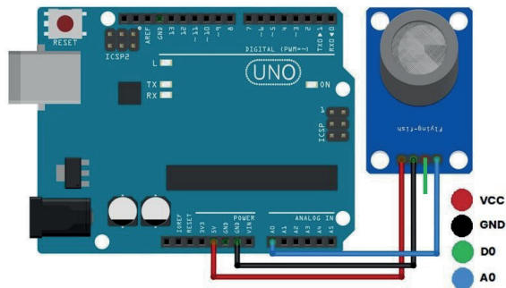
Figura 3. Sensor MQ-6. Conexión salida Analógica, (MQ-6 Detector de Gas LP - UNIT Electronics
