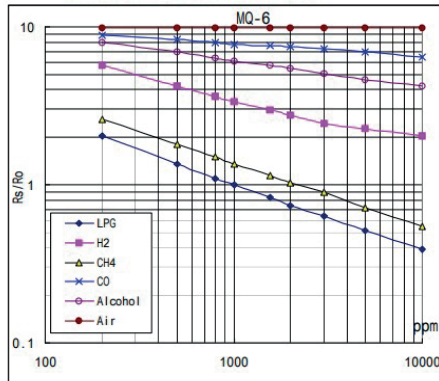
Figura 2. Características de sensibilidad del MQ-6
