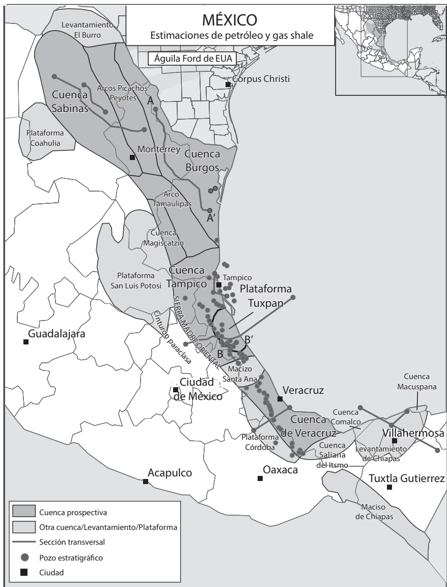
Mapa IV.2. Cuencas de gas de lutitas en tierra en el noreste de México
