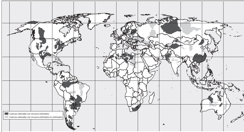
Mapa IV.1. Cuencas de formaciones de aceite y gas de lutitas
